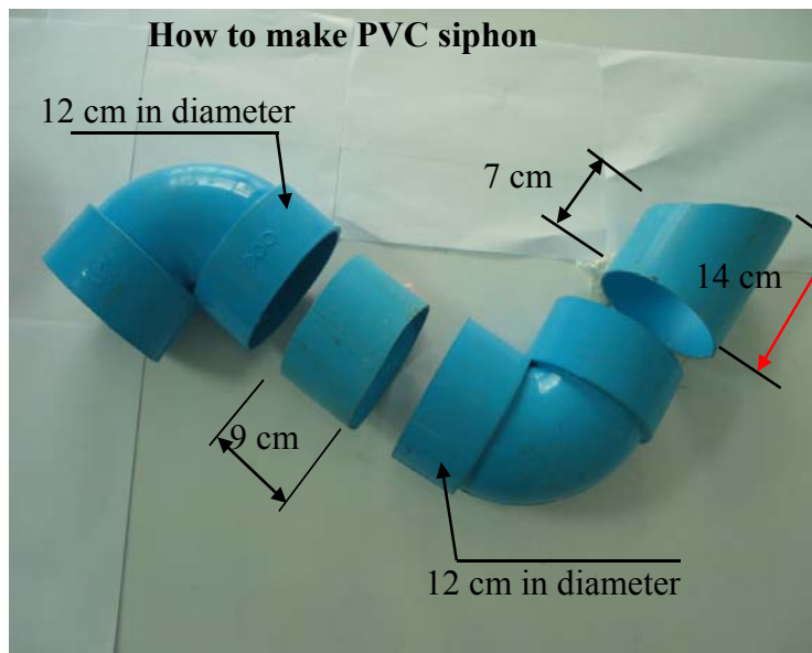
Fig 12: PVC siphon
