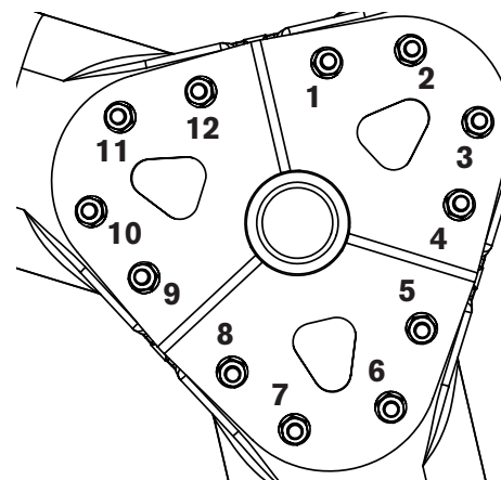
Séquence de serrage des boulons des pales
