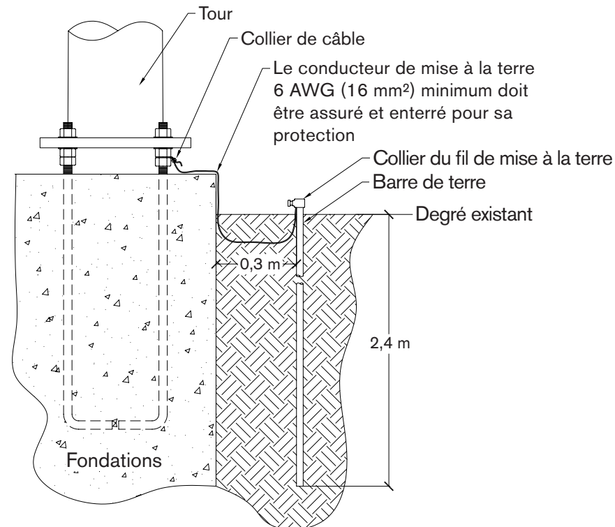
III. 1 Électrode enfoncée dans le sol.
