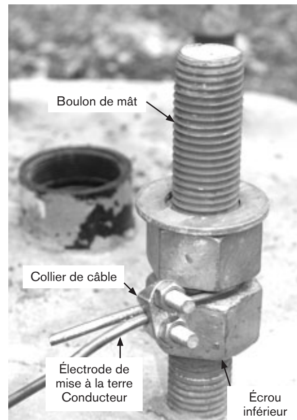
III. 3 Boulon des fondations du mât.
