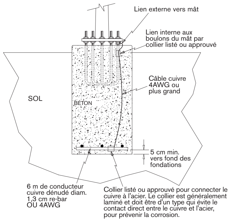
Fig. 4 Électrode enchâssée dans le béton.
