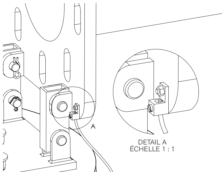
III. 2 Attacher le fil de terre à la base du mât.
