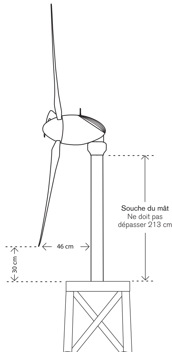
Distances minimales par rapport aux pales
