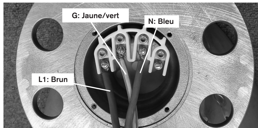
III. 3 Disposition des fils à la connexion du dispositif d'orientation (230V, 50Hz, monophasé).
