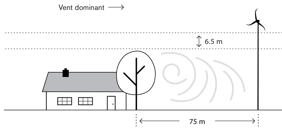
Emplacement optimal du Skystream.
